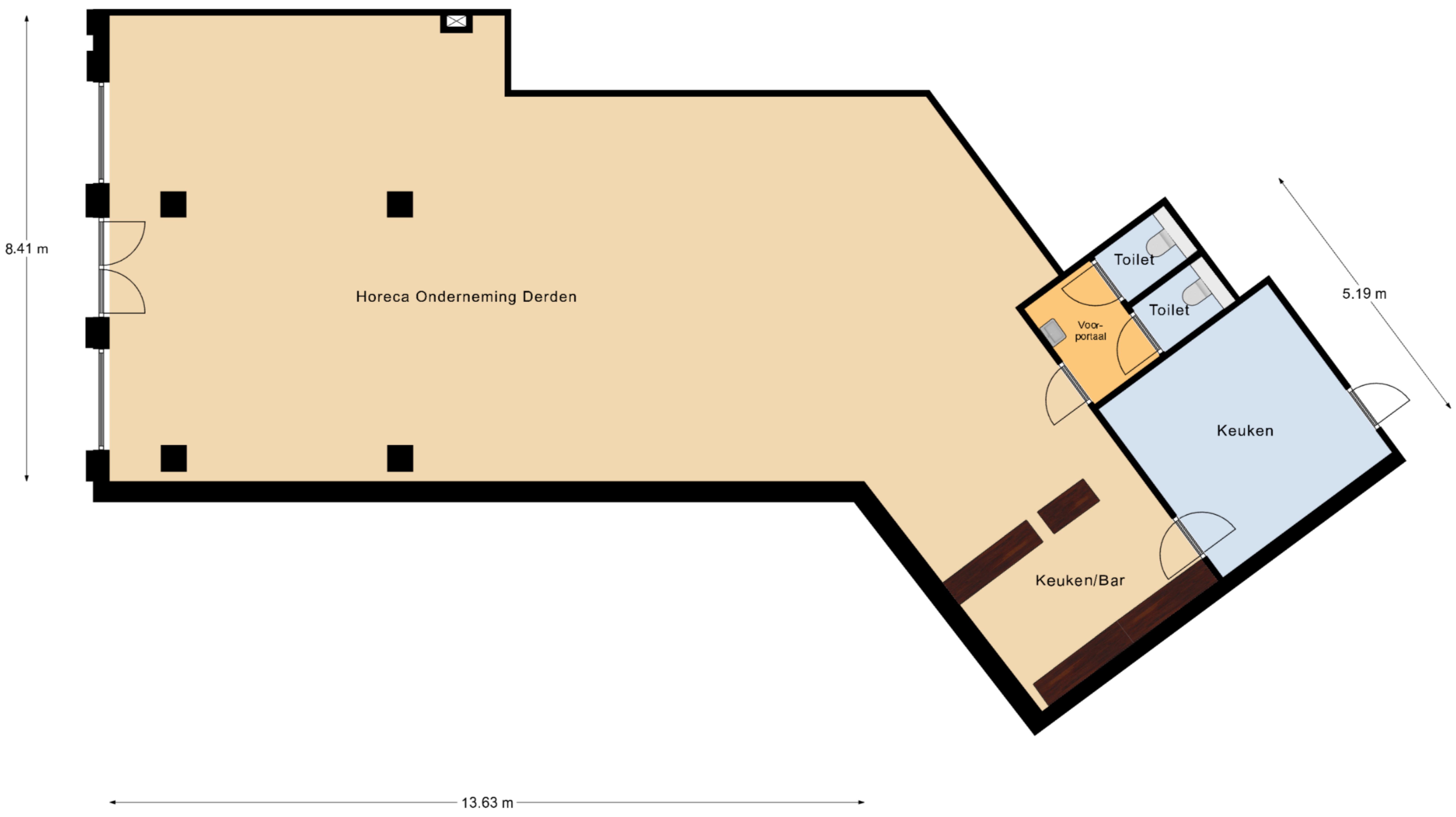
Plattegrond
