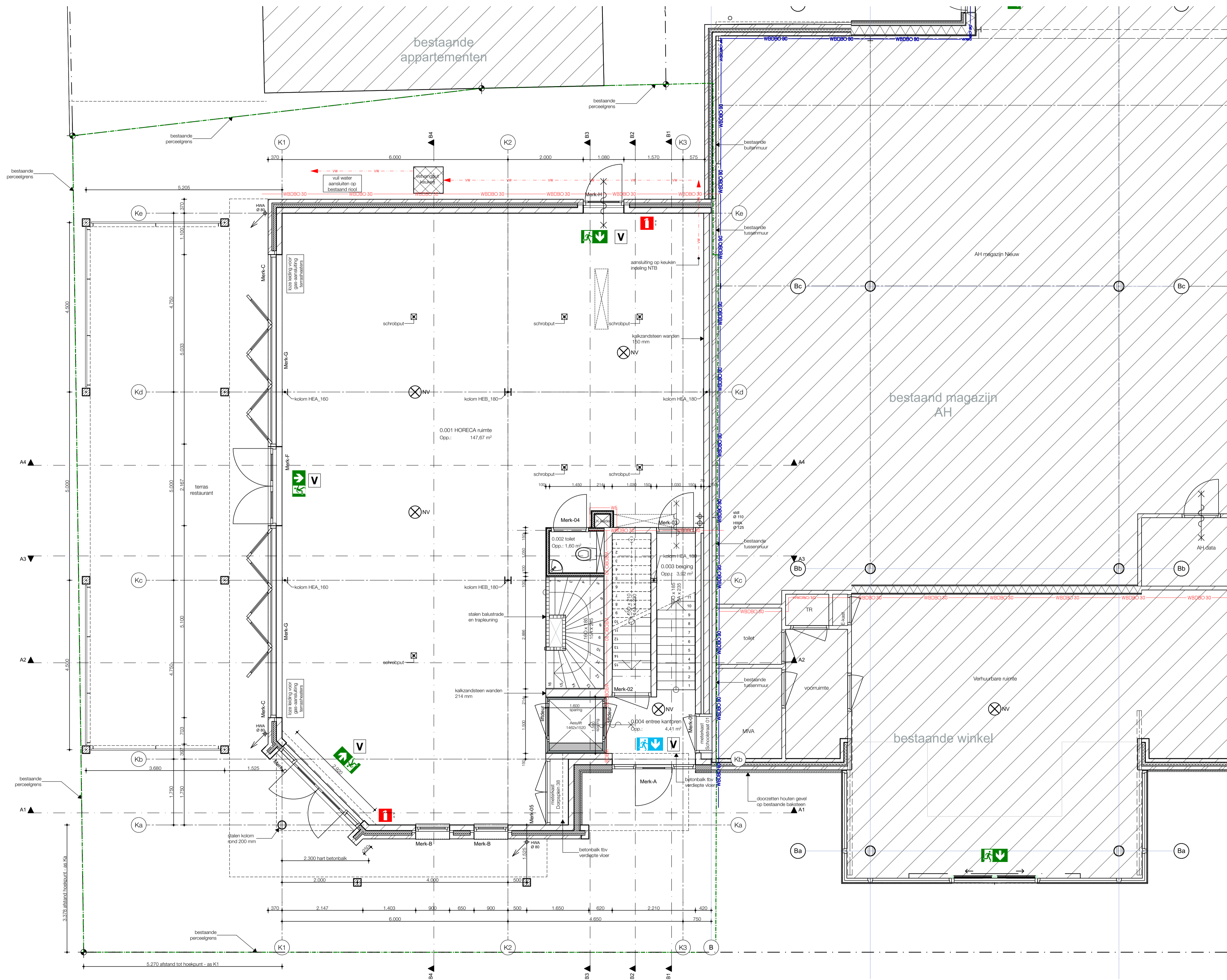
Begane grond
